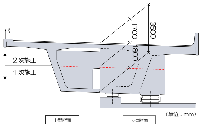
図-6 分割位置図(対策後)
