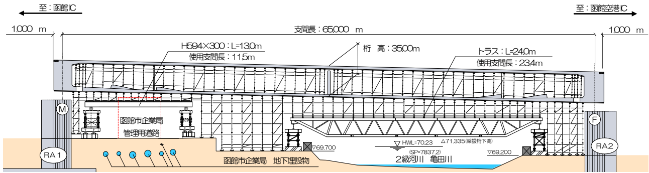
図-11 R橋(上り線)支保工側面図
