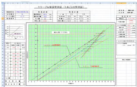
図-15 緊張管理画面
