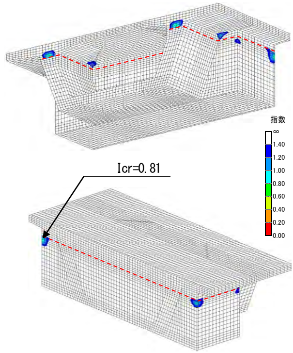
図-5 最小ひび割れ指数の分布(標準案)
