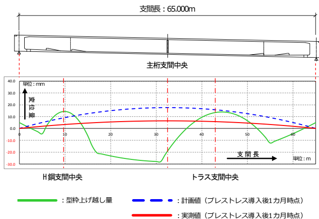
図-12 主桁変位量・上げ越し量
