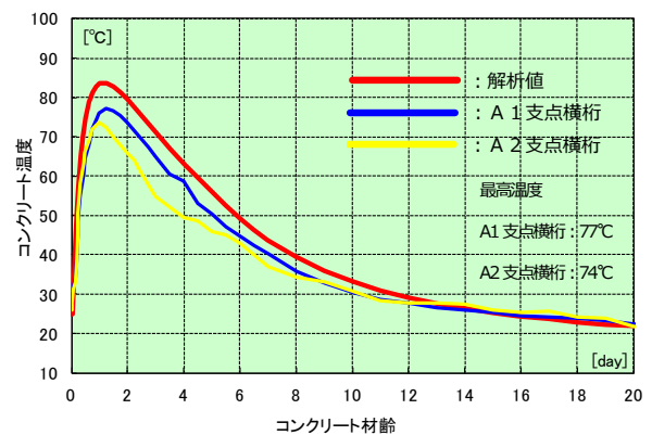
図-10 温度測定結果（2次施工）
