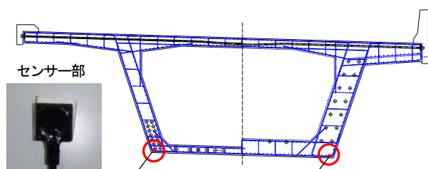
図-18 充填検知センサー配置図
