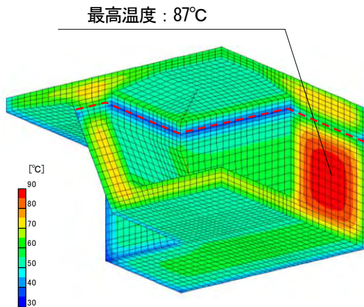
図-4 温度分布(標準案)
