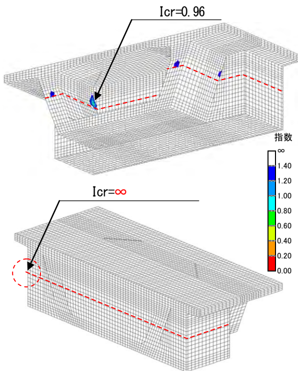
図-8 最小ひび割れ指数の分布（対策後）
