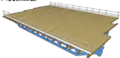
図-20 3Dモデル
