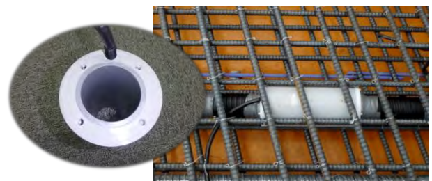
図-13 磁歪式張力センサー
