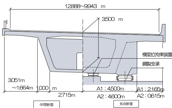
図-1 R橋（上り線）断面図
