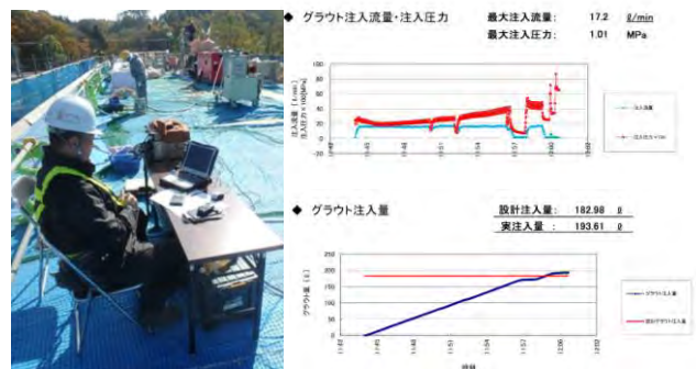
図-16 注入管理システムによる注入管理
