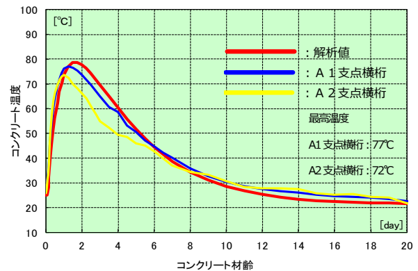
図-9 温度測定結果（1次施工）
