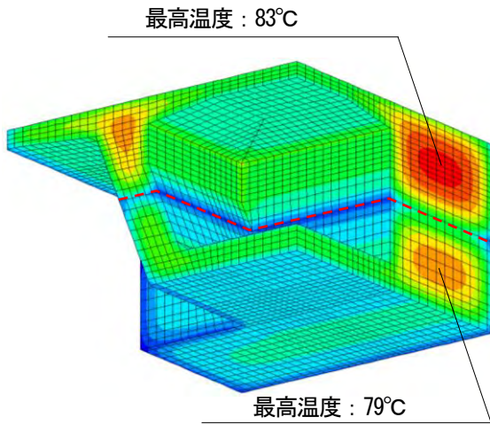
図-7 温度分布（対策後）
