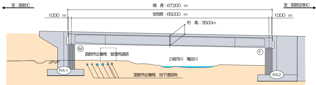
図-2 R橋（上り線）側面図
