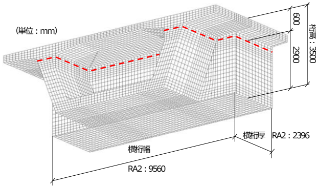
図-3 支点横桁モデル(標準案)
