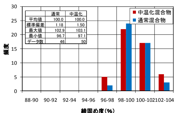
図-1 締固め度（ストアス混合物）
