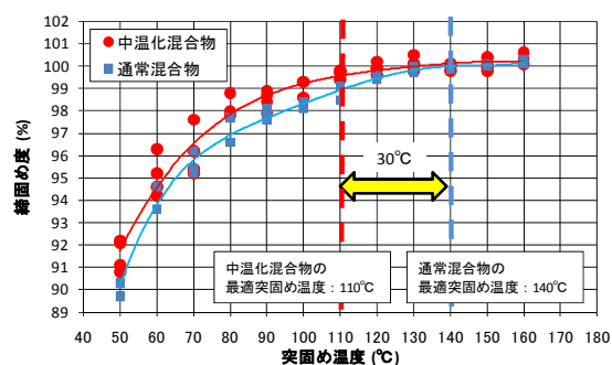
図-9 マーシャル安定度試験結果（発泡系）
