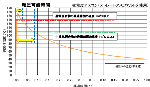
図-17 中温化混合物の転圧可能時間
