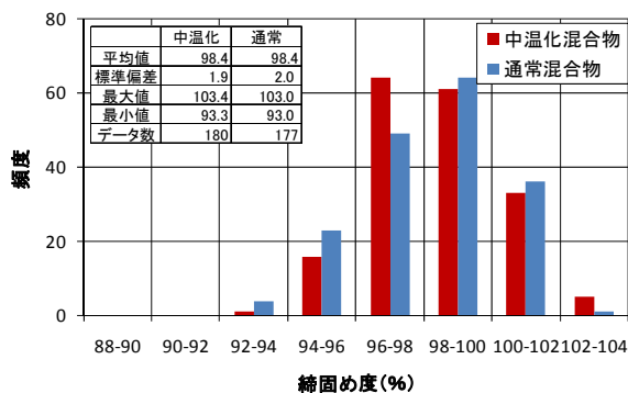
図-2 締固め度（改質 As 混合物・Ⅰ型）
