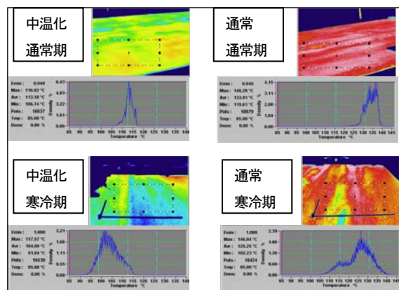
図-21 寒冷期及び通常期施工の敷均し時の温度分布
