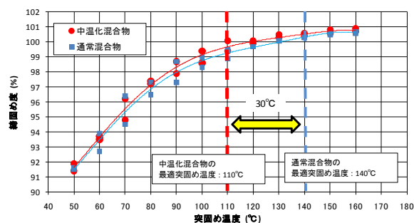
図-11 マーシャル安定度試験結果（滑剤系）
