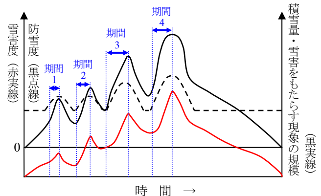
図-9 積雪量と防雪度、雪害度との関係 中村 16) を改変 雪害度 = 積雪量・雪害をもたらす現象の規模 - 防雪度 期間 1 から期間 4 は、表-4 を参照
