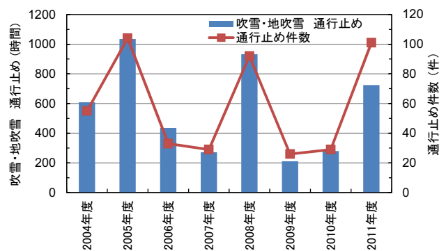
図-5 通行止めの累計時間と件数（吹雪・地吹雪） 8)-15)
